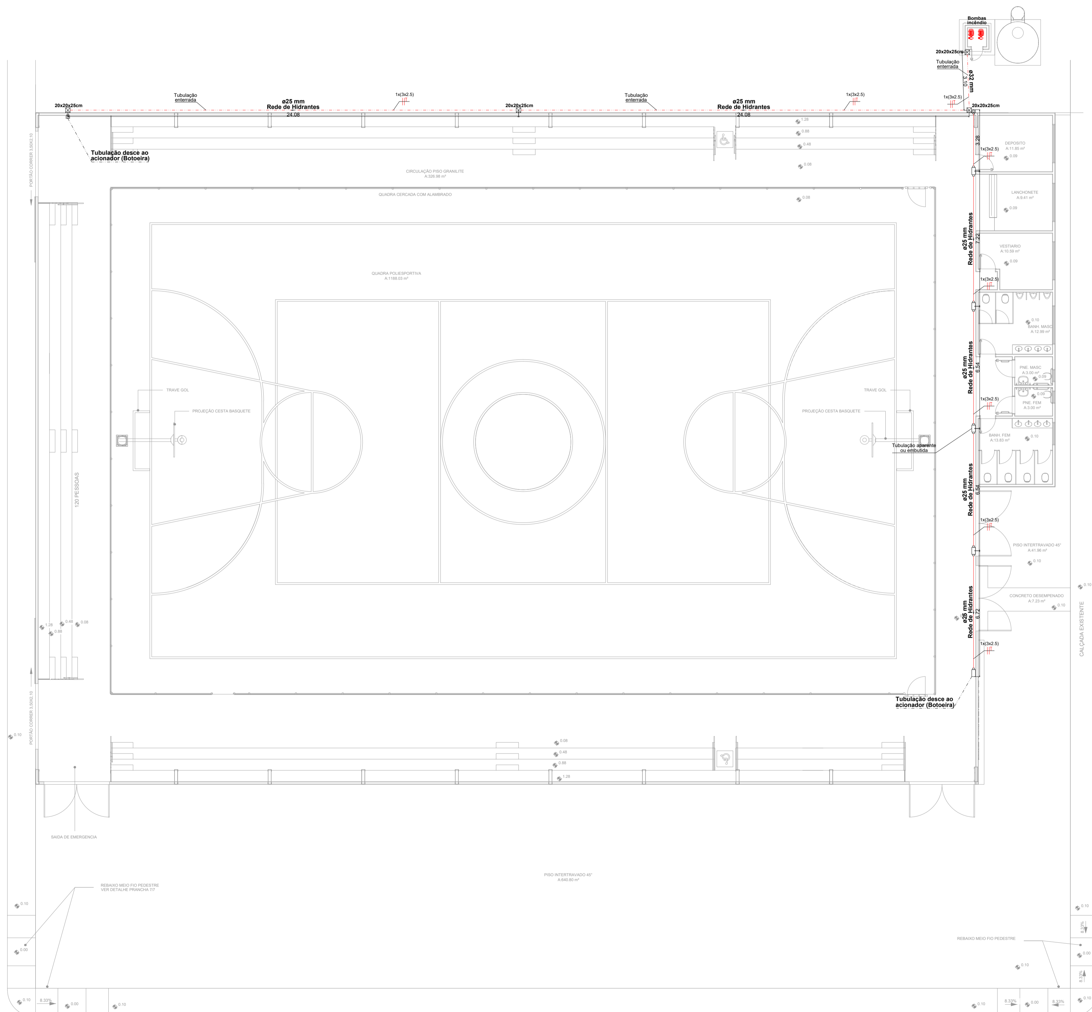
1 Planta baixa - Infraestrutura rede de hidrantes ESCALA: 1:125
