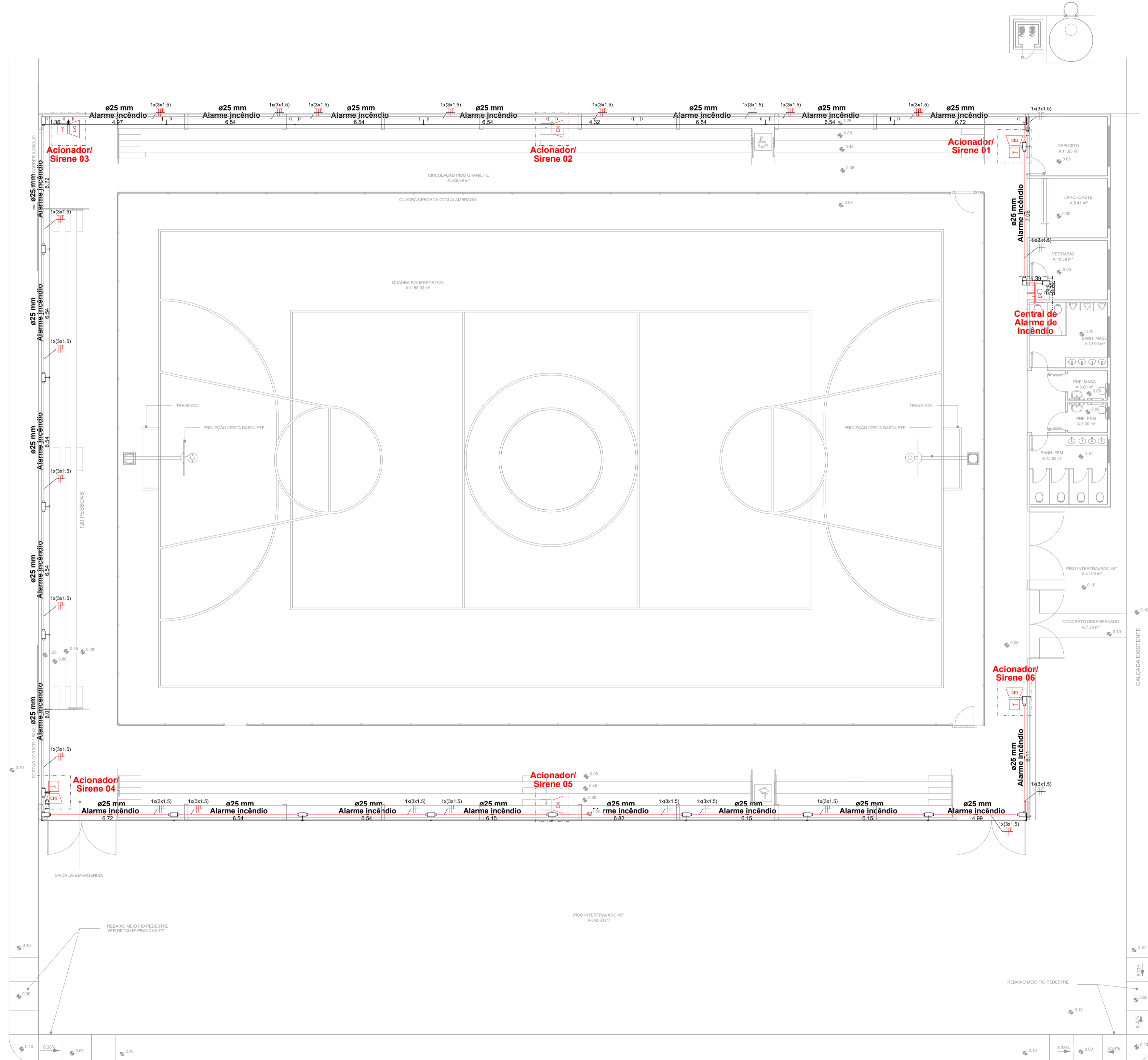
1 Planta baixa - Alarme de Incêndio ESCALA: 1:125
