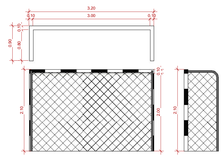
DET. GOL 1:50
