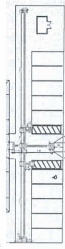
5 COBERTURA CASA DE MÁO. 1:25
