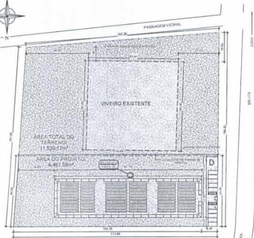
2 PLANTA DE LAYOUT 1:200
