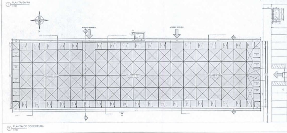
2 PLANTA DE COBERTURA 1:100
